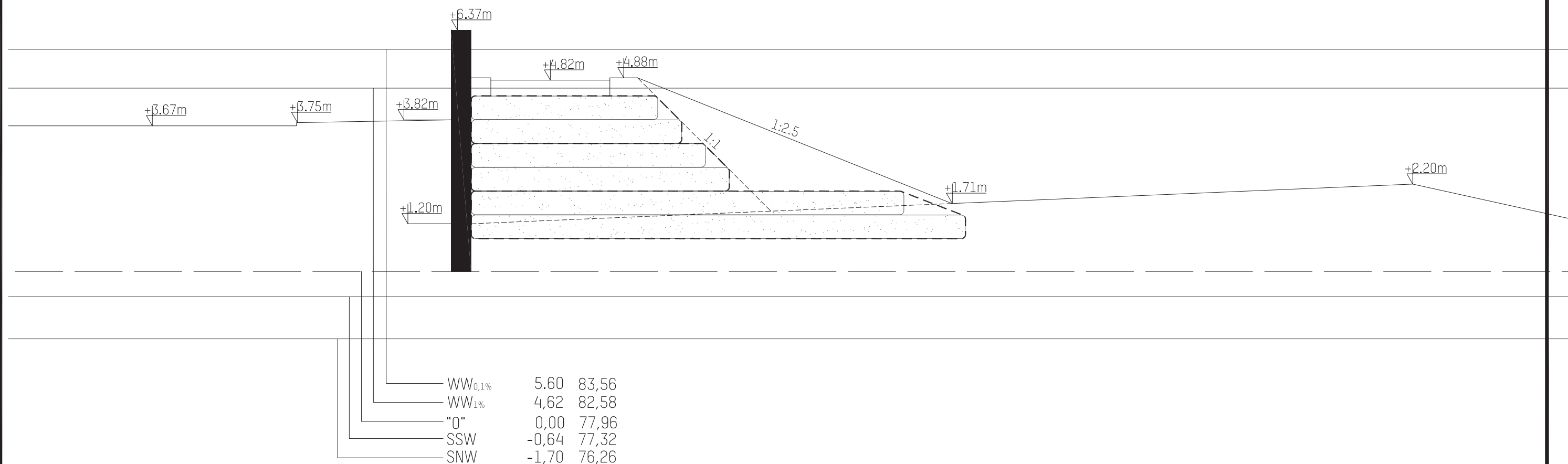
PRZEKRÓJ CHARAKTERYSTYCZNY NA OSI WĘZŁA Z ULICĄ GWIAZDZISTĄ (520KM WISŁY) SKALA 1:100
