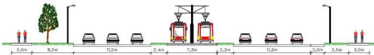
Rys. 2.5 Typowe rozwiązanie przekroju poprzecznego na ul. Puławskiej od „przejścia” trasy tramwajowej w oś do skrzyżowania z ul. Poleczki
