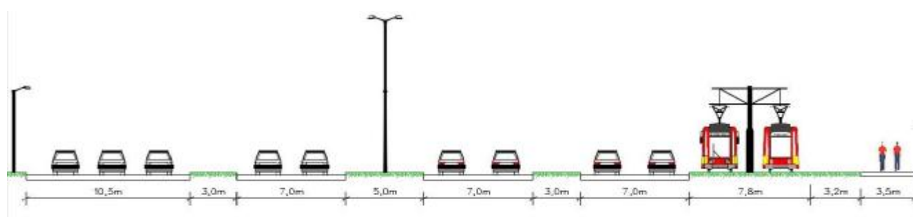
Rys. 2.3 Typowe rozwiązanie przekroju poprzecznego na ul. Puławskiej w rejonie Torów Wyścigów Konnych.
