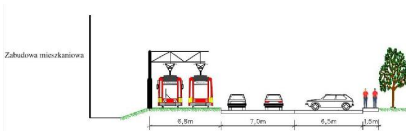
Rys. 2.8 Typowe rozwiązanie przekroju poprzecznego na ul. Wojska Polskiego od ul. L. Okulickiego do ul. Nadarzyńskiej
