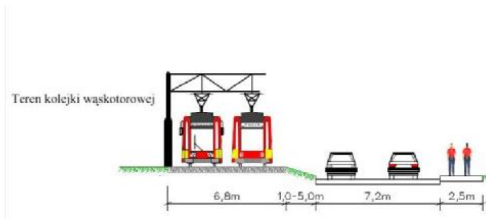
Rys. 2.9 Typowe rozwiązanie przekroju poprzecznego na ul. H. Sawickiej od ul. Nadarzyńskiej do ul. Sienkiewicza
