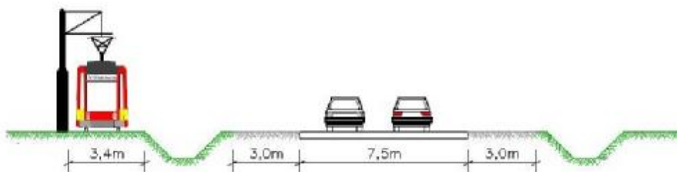
Rys. 2.14 Typowe rozwiązanie przekroju poprzecznego na ul. Armii Krajowej
