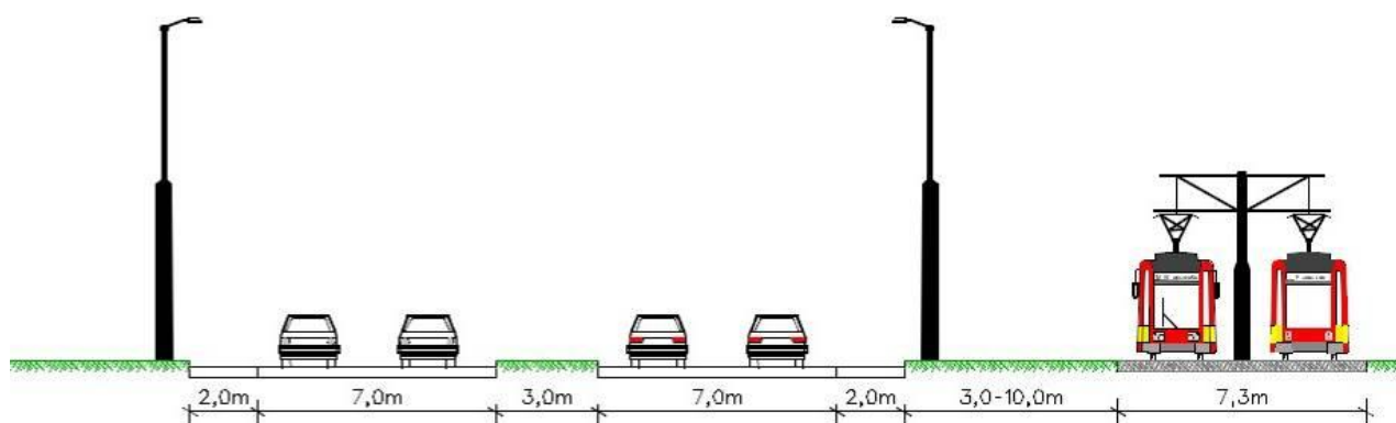
Rys. 2.7 Typowe rozwiązanie przekroju poprzecznego na ul. Puławskiej od skrzyżowania z ul. Karczunkowską do ul. Okulickiego
