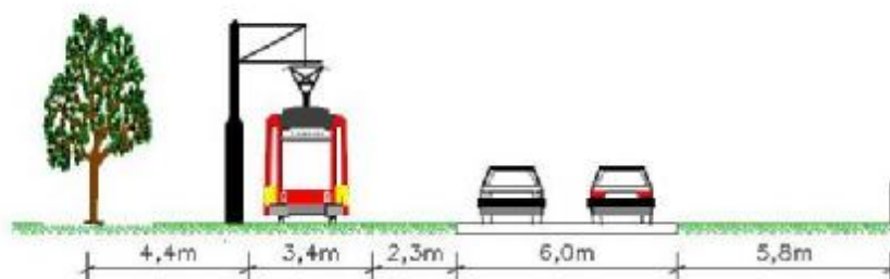
Rys. 2.11 Typowe rozwiązanie przekroju poprzecznego na ul. Okulickiego od ul. Wojska Polskiego do ul. Powstańców Warszawy
