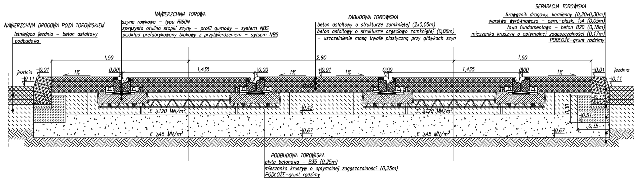
Rys. 4.1 Przekrój konstrukcji bezpodsypkowej w systemie NBS – wersja z zabudową z betonu asfaltowego. Możliwa zabudowa tłuczniem i humusem z porostem trawiastym
