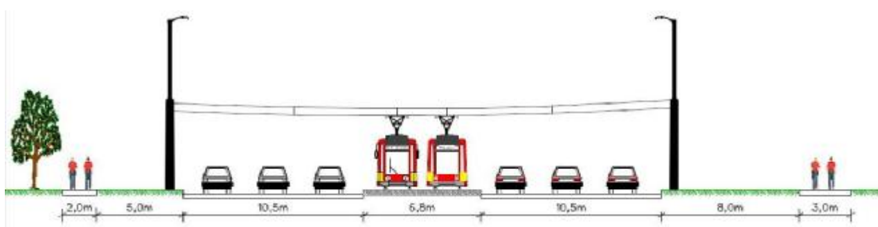
Rys. 2.6 Typowe rozwiązanie przekroju poprzecznego na ul. Puławskiej od skrzyżowania z ul. Poleczki do ul. Karczunkowskiej
