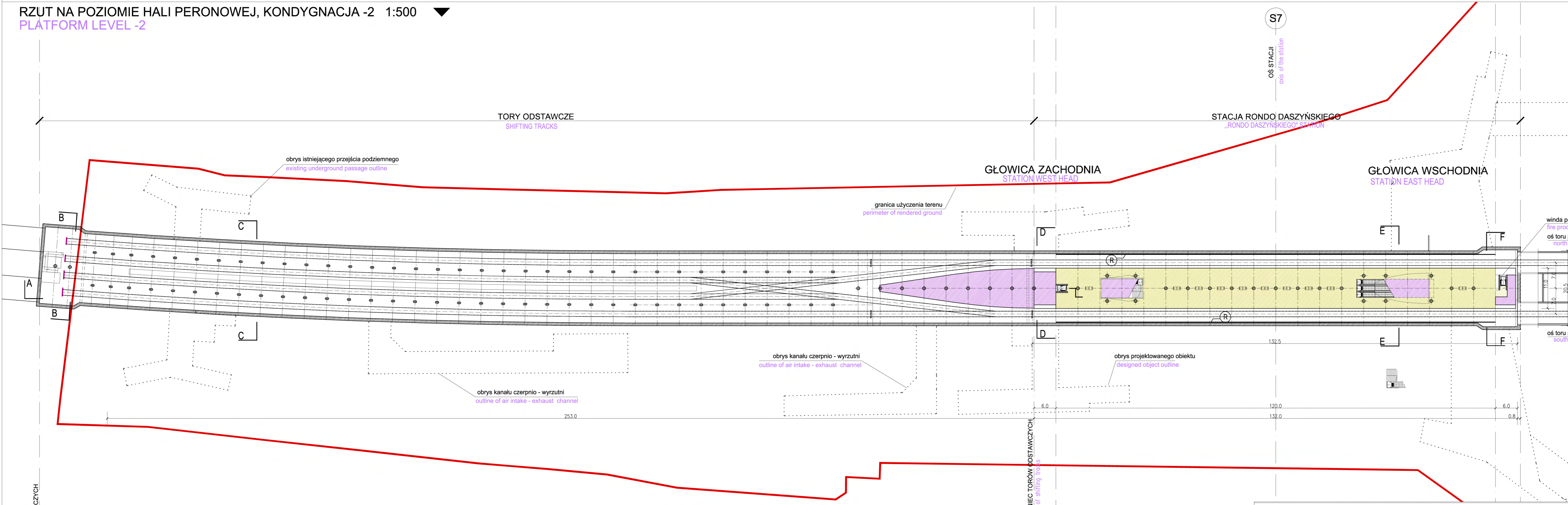
RZUT NA POZIOMIE HALI PERONOWEJ, KONDYGNACJA -2 1:500 PLATFORM LEVEL -2
