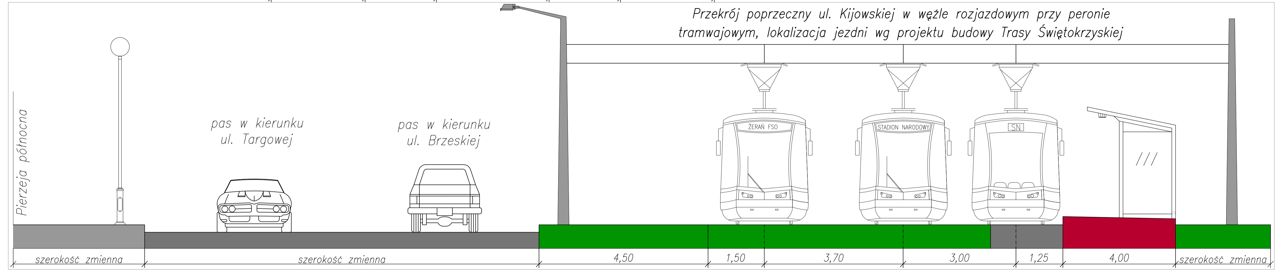
Przekrój poprzeczny ul. Zielenieckiej przy peronie tramwajowym przystosowanym do obsługi imprez masowych
